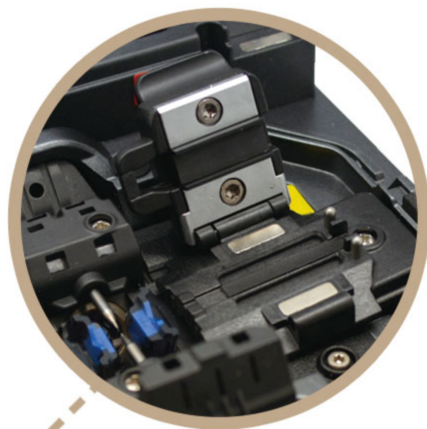
Universal Holder - 250µm - 900µm - 2~3Ø - Indoor
